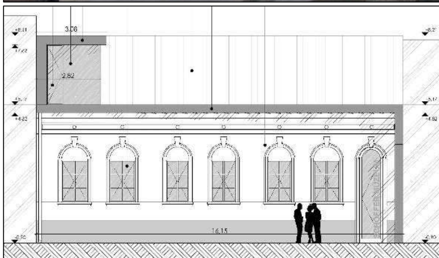
2012-es átépítés homlokzatterve
